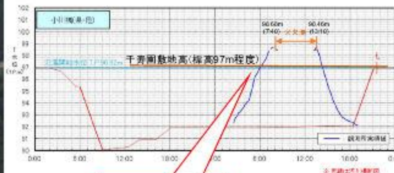
小川の水位(本川合流部より約0.1km) ※熊本県の危機管理型水位計
